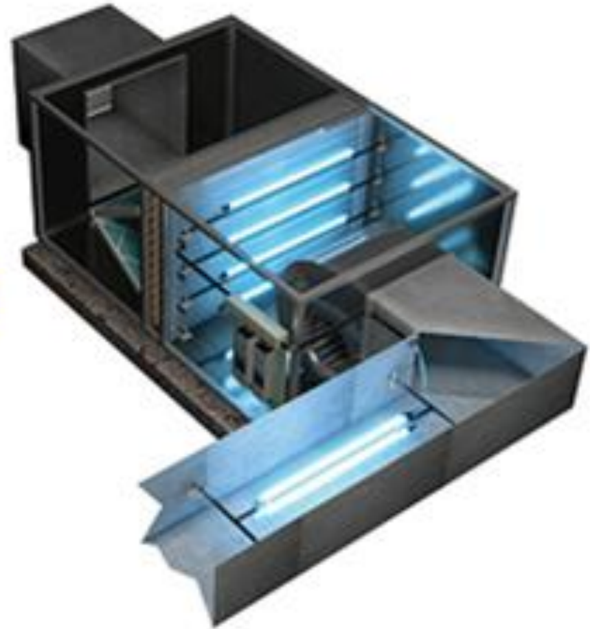
Bi-Polar Ionization
